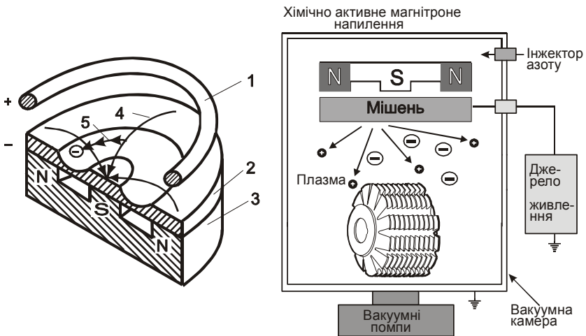
Рисунок 5 – Схема магнетронного розпилення:
