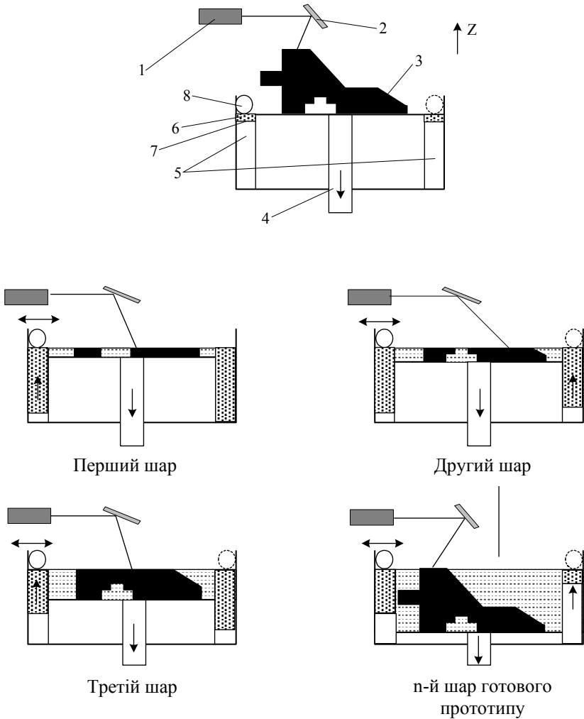
Рисунок 7 – Схема одержання тривимірного твердотільного виробу пошаровим нарощуванням вибірним лазерним спіканням: 1 – лазер, 2 – оптична система, 3 – готовий виріб, 4 – рухлива (по осі Z) робоча платформа, 5 – бункери для подачі порошкового матеріалу, 6 – порошковий матеріал, 7 – рухливий стіл бункеру, 8 – ролик для подачі порошку та вирівнювання шару
